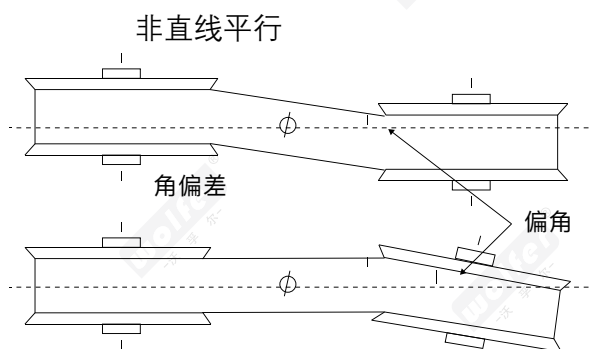
图1 皮带轮不对称图示
