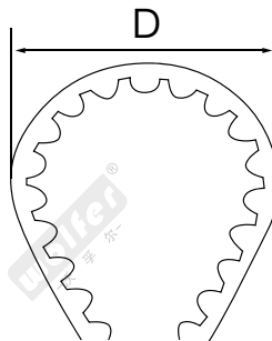
图 2 同步带的最小弯曲直径
