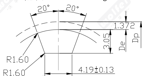
H型齿形图
