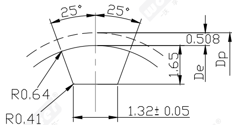
XL型齿形图
