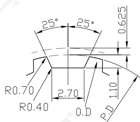
AT5型齿形图
