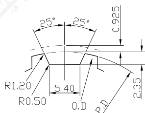
AT10型齿形图
