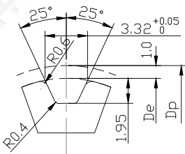
T5型齿形图
