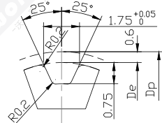
T2.5型齿形图
