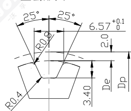
T10型齿形图
