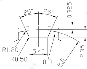
AT10型齿形图
