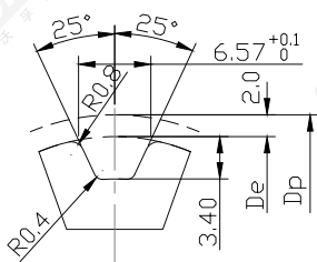
T10型齿形图
