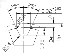
T5型齿形图
