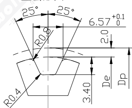
T10型齿形图
