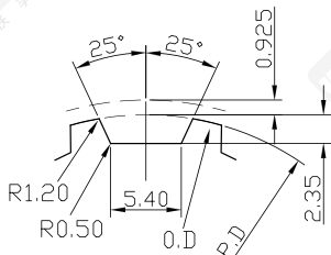
AT10型齿形图
