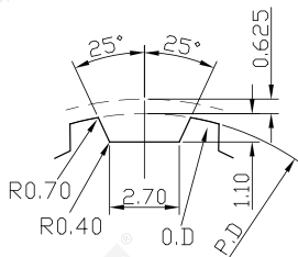
AT5型齿形图
